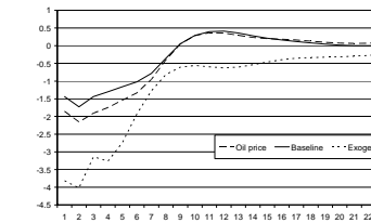
B) Variables
