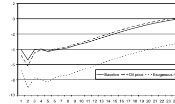
B) Variables
