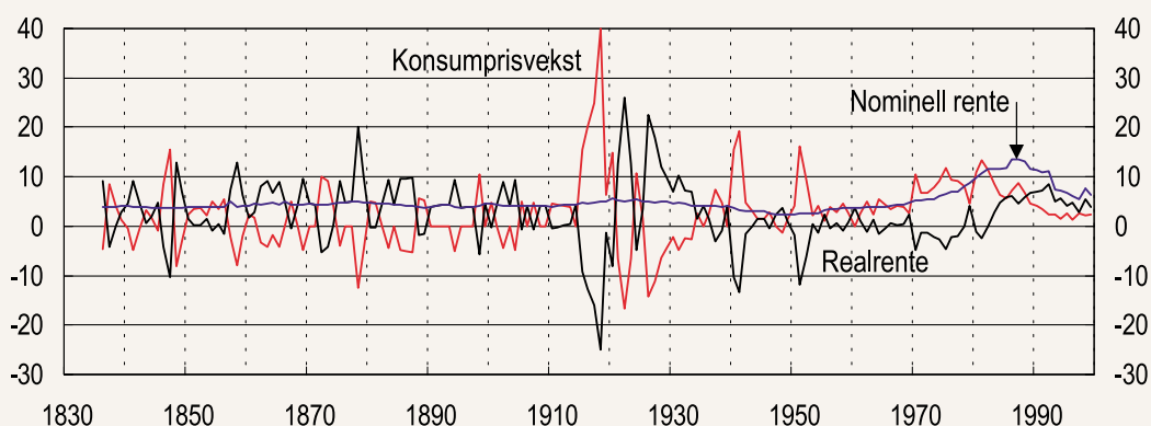
Figur 2 Realrentenivå 1836 - 1999
